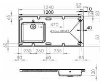
Coupe A-A Echelle 1 : 20
